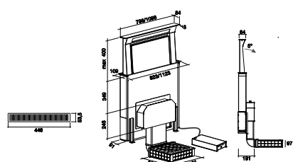
Umluftbetrieb mit flachem Motor u. Umluftbox
